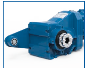
Schumpfscheibe und Drehmomentstütze
